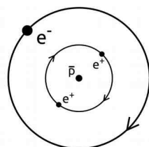
\bar{H}^+ et e^- Stable ?
